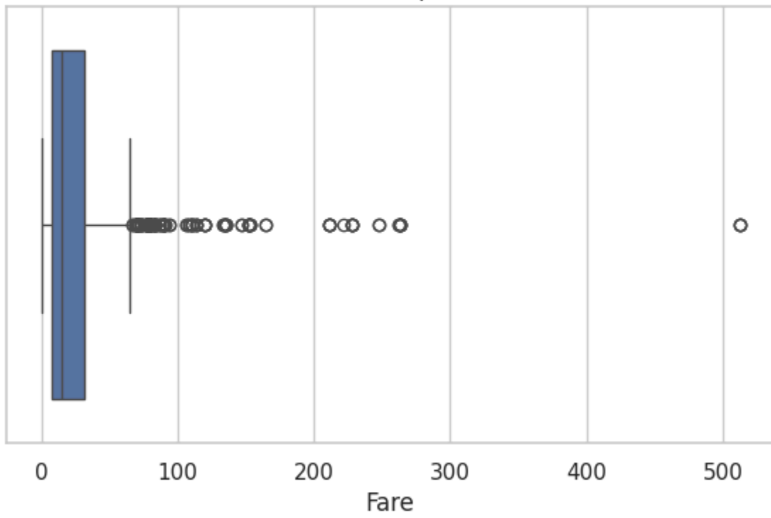
Fare Boxplot
